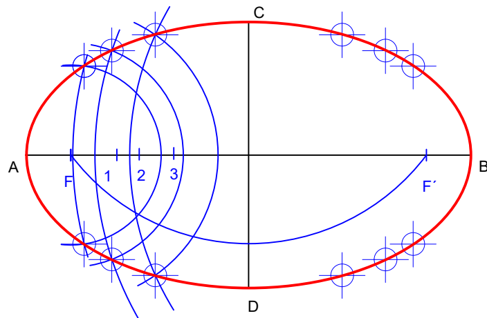
1- Construcción de una elipse por puntos
