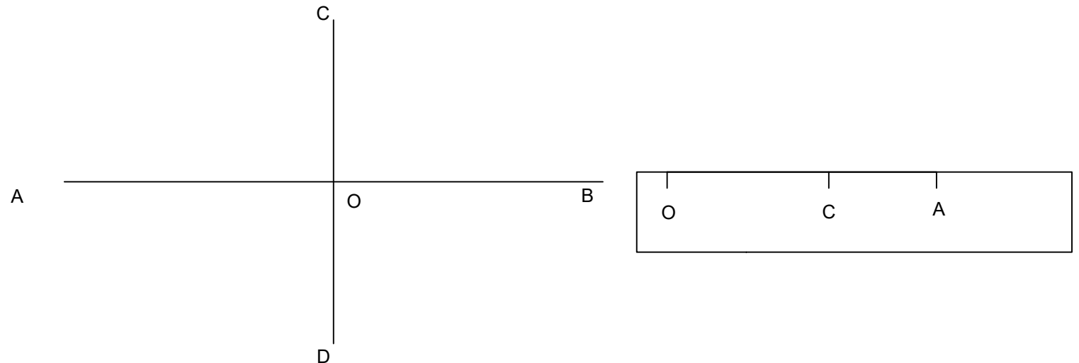
3- Construcción de una elipse por el método de la tarjeta
